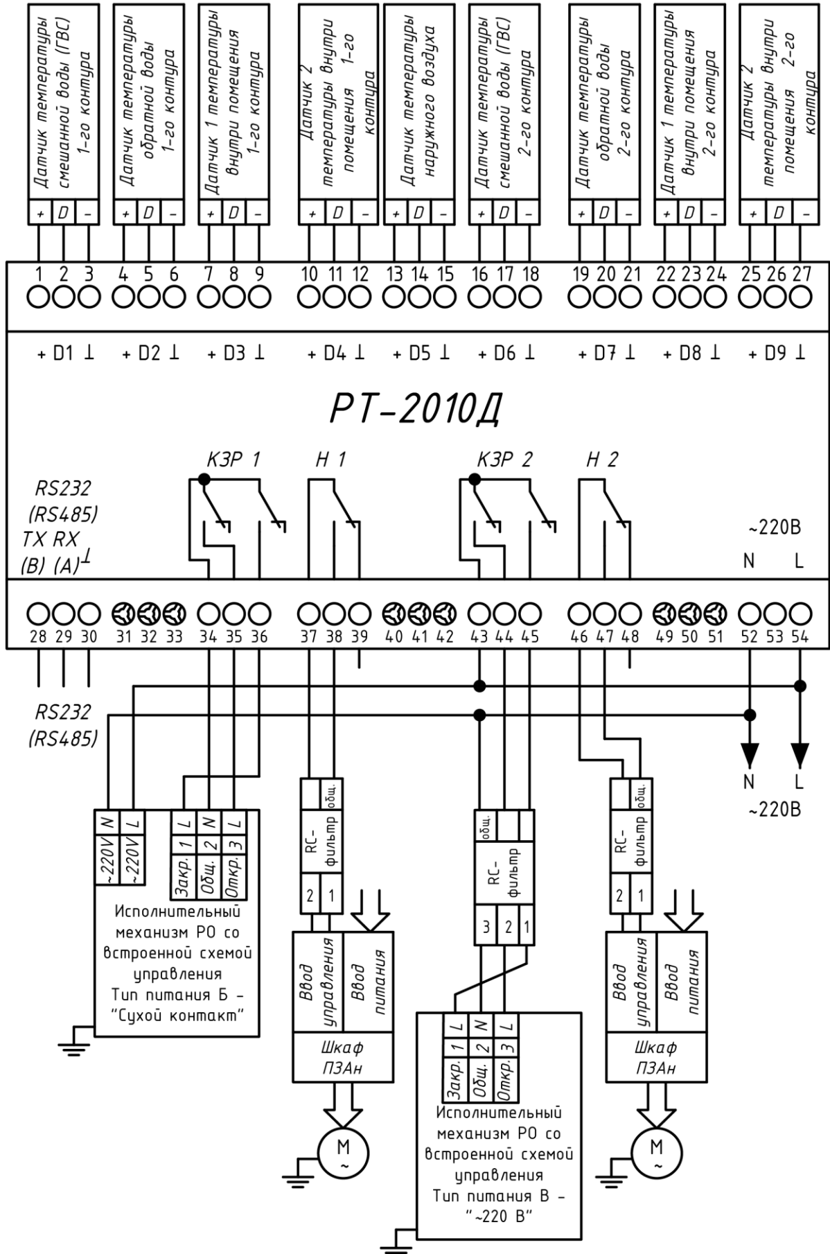
Схема электрическая подключений (ИМ с напряжением 220 В)
