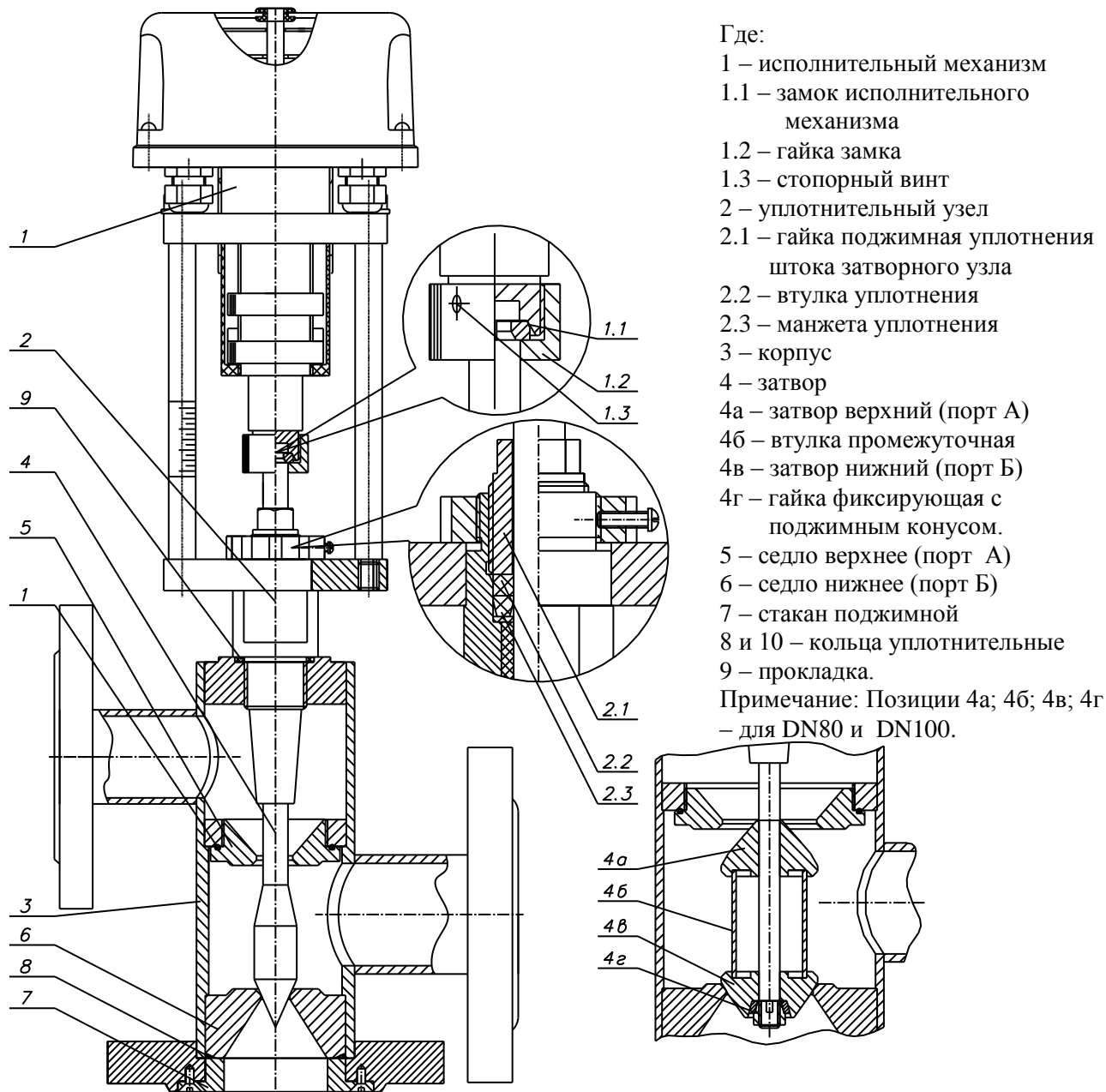
Рисунок 1. Общее устройство клапана смешивающего трехходового КСТ-XX(X)/XX.X-XX
