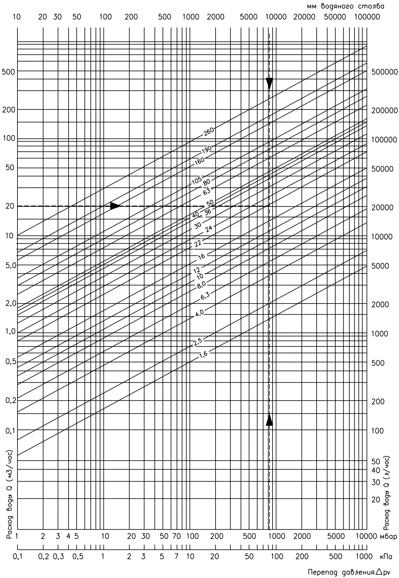
Диаграмма1: Kvs, определение размера, рабочая среда – вода
