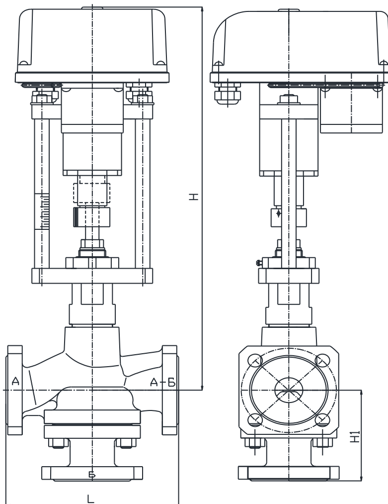
Рисунок 1. Общий вид клапана
