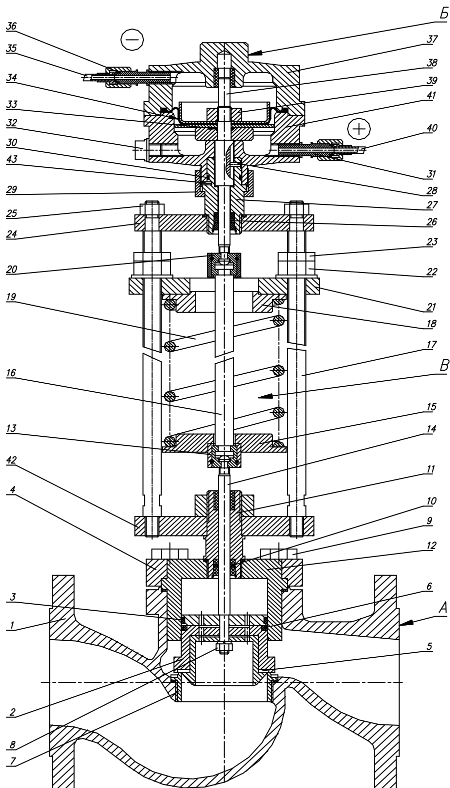
Рисунок 1. Общее устройство регулятора РД-В-65.
