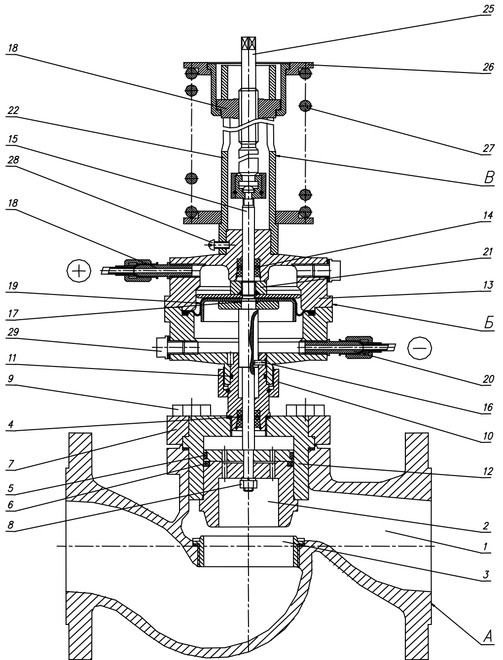
Рисунок 1. Общее устройство регулятора РД-А-65.
