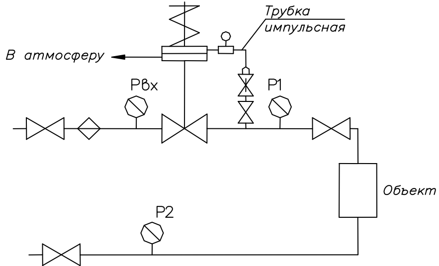
Рисунок 1. Схема подключения регулятора давления (РД-А).
