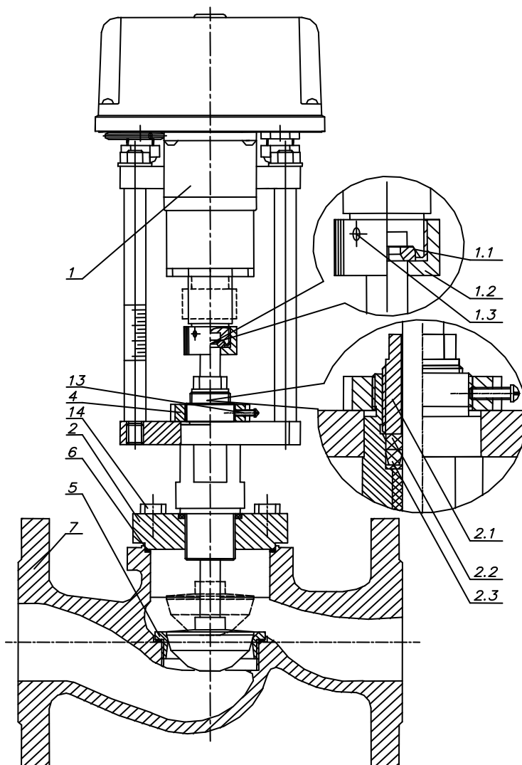
Рисунок 1. Общее устройство клапана КЗР - 40/XX.Б-XX
